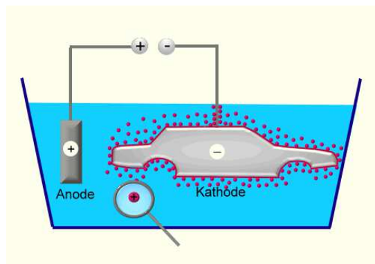
Abbildung 2. Schematische Darstellung des E-Coating-Verfahrens
